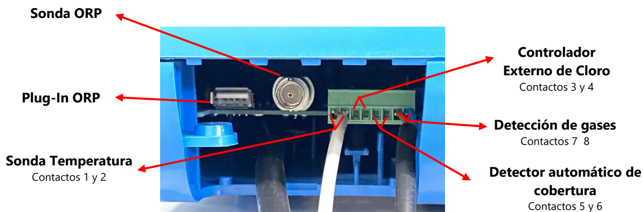
Figura 6 - Conexiones internas
